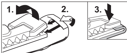
12. ábra: A felmosórongy rögzítése
