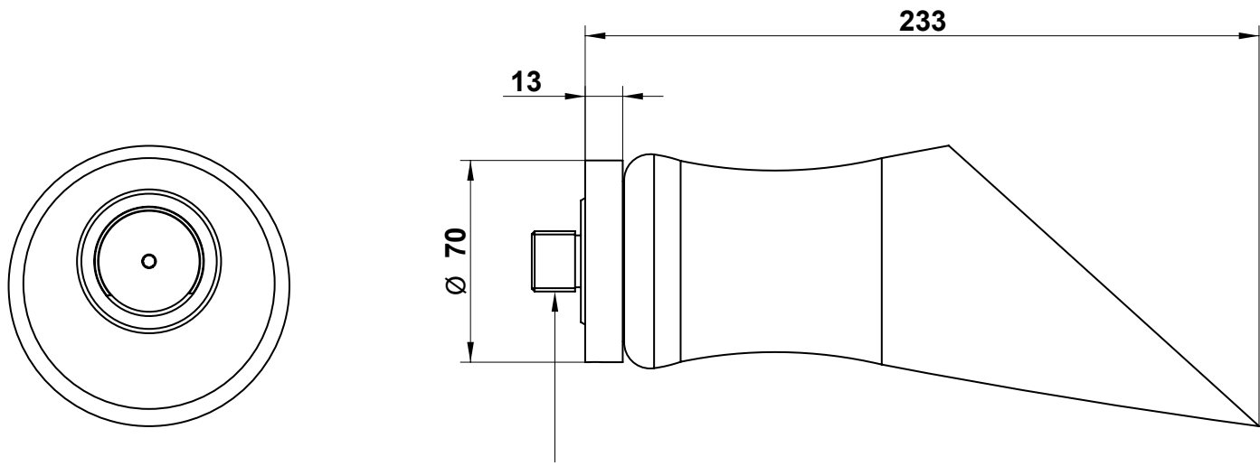
ATTACCO 1/2" GAS M.
