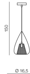
Gordon 1 AZ2166 G9 1x MAX 33W metal/glass
