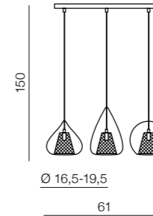
Gordon Mix Line AZ2168 G9 3x MAX 33W metal/glass
