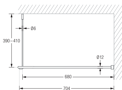
DR700HD Seitenansicht:
