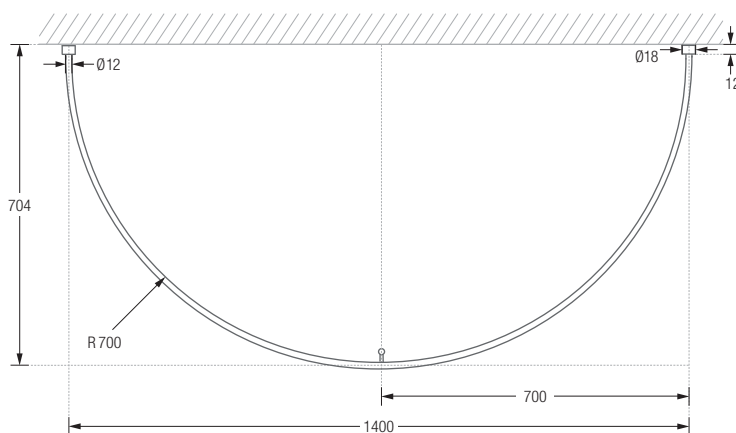
DR700HD Draufsicht:
