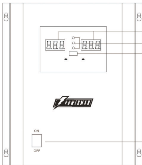
Передняя панель
