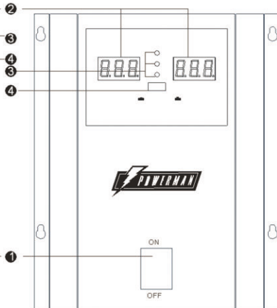
Передняя панель
