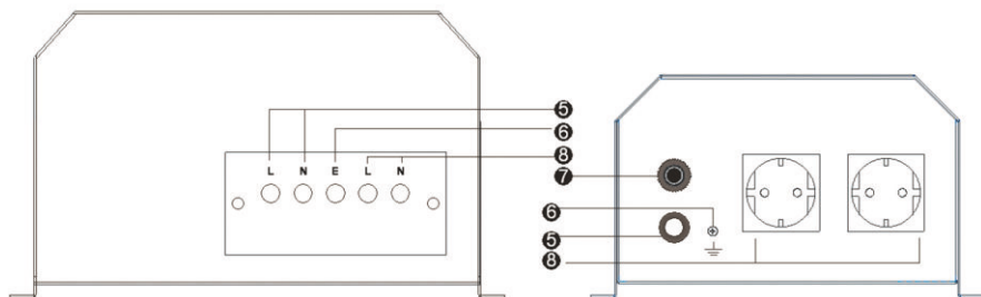
Панель подключения
