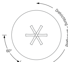
GSTH10F-B / GSTH10FE-B Draufsicht:
