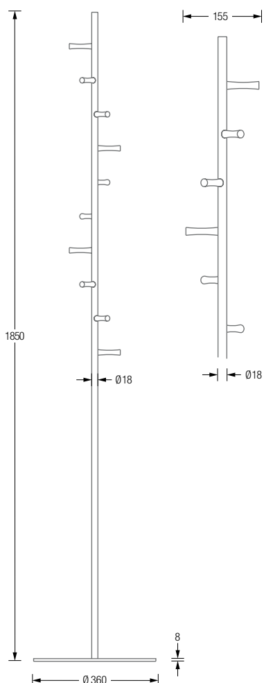
GSTH10F-B / GSTH10FE-B Seitenansicht:
