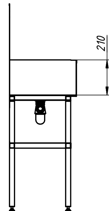
A-A (1:14)
