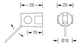
Winkelflexible Wandbefestigung:
