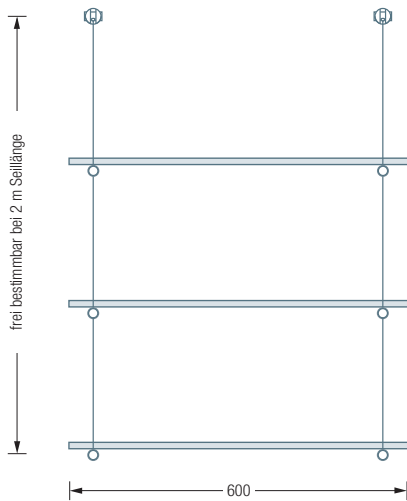
RST260-3-B Frontansicht:
