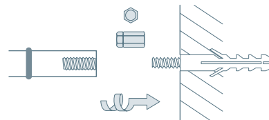
Wandmontage Glasbodenträger:
