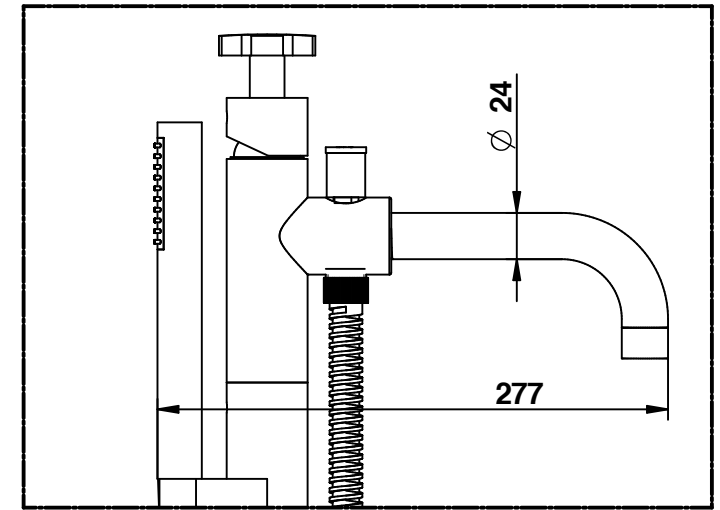
DETTAGLIO A
