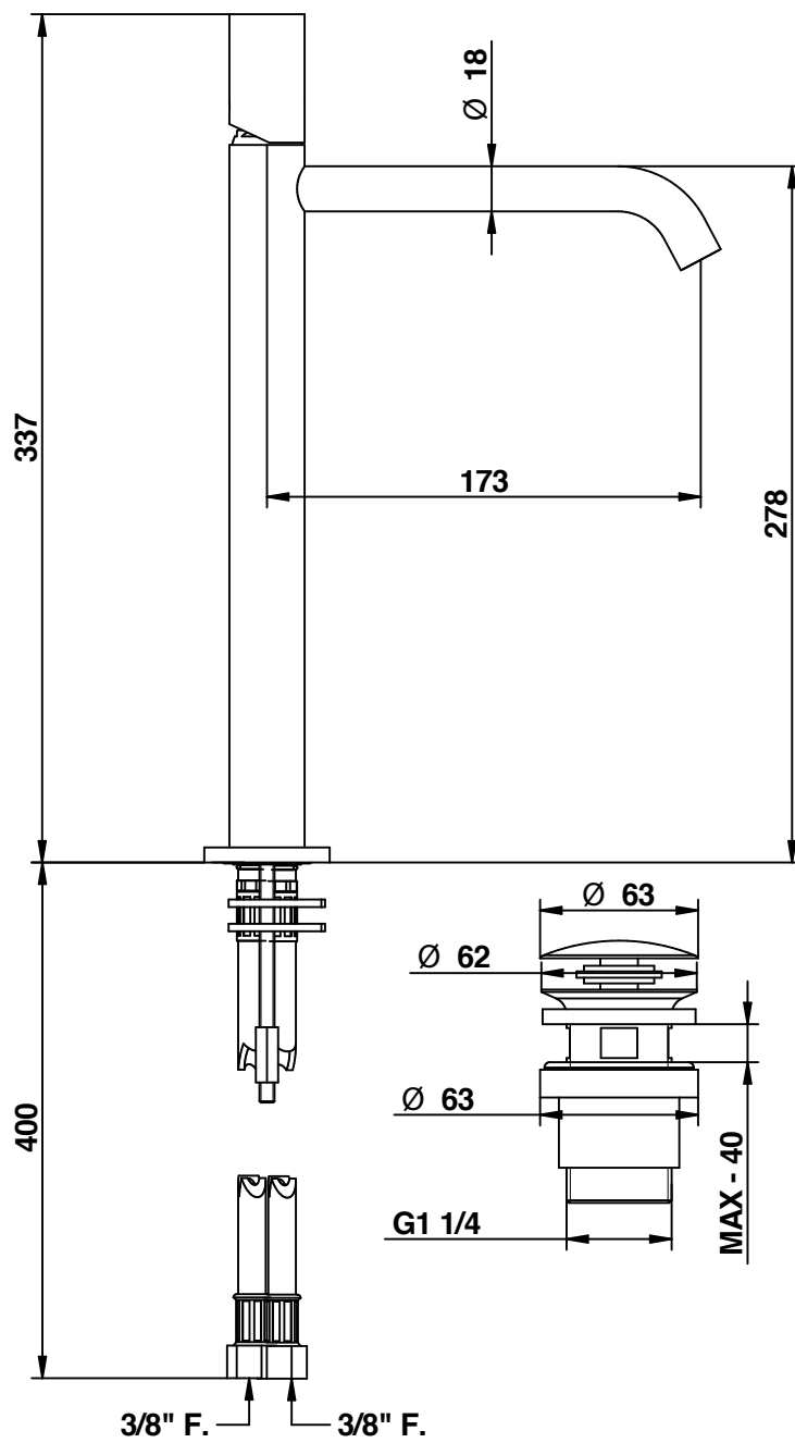
Miscelatore lavabo alto con piletta clic - clac
