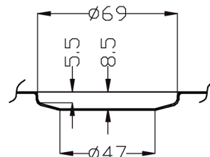
C-C 4:1
