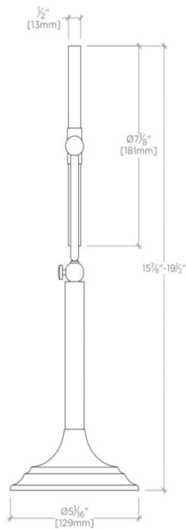
SIDE VIEW SCALE: 3"=1'-0"
