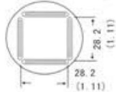
A1129 QFP14X28 (1.1X1.1)
