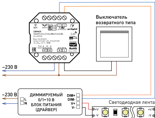
Рисунок 1. Схема подключения диммера SMART-D14-TUYA-DIM-PUSH-IN
