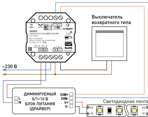
Рисунок 2. Схема подключения диммера SMART-D14-TUYA-DIM-PUSH-IN с использованием выхода AC OUT
