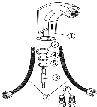
Установочная схема №1
