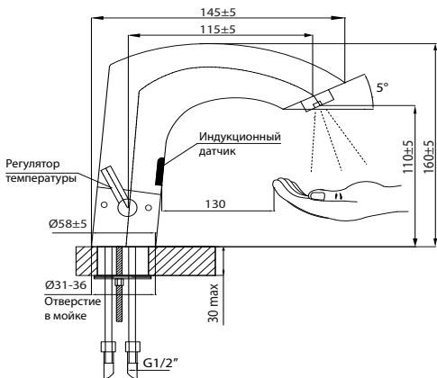
Установочная схема №1
