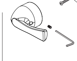
RP100978 ▲ Handle Kit Juego de herrajes de la Manija Manette en kit
