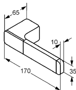
Размеры
