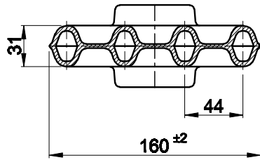
A-A KESİTİ
