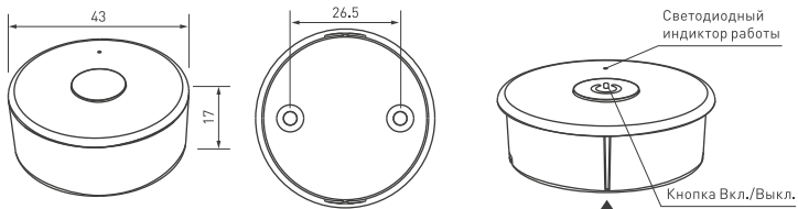
Рис. 1. Конструктивный чертеж.
