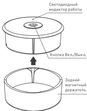
Рис. 2. Схема установки.
