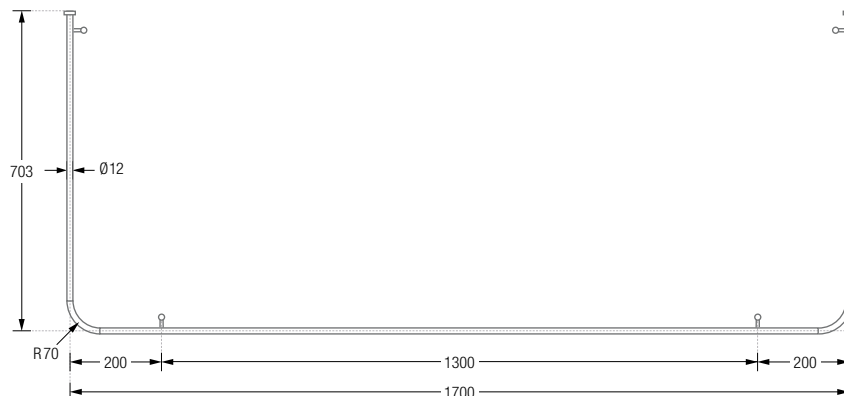
Produktbeispiel DSU1700-700F Draufsicht:
