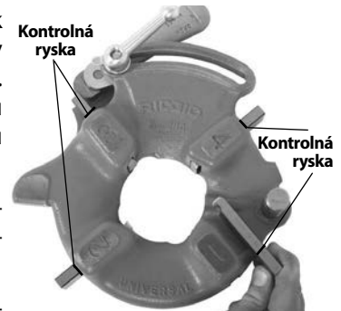
Obrázok 8 – Vkladanie závitorezných čelustí
