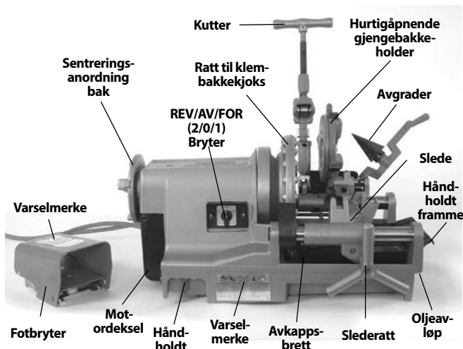
Figur 1 – 300 Compact gjengemaskin
