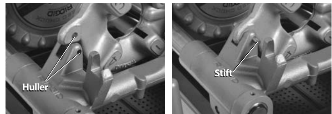
Figur 26 – Fastgørelse af venstreskærehovedet
