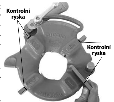
Obrázek 8 – Vkládání matic
