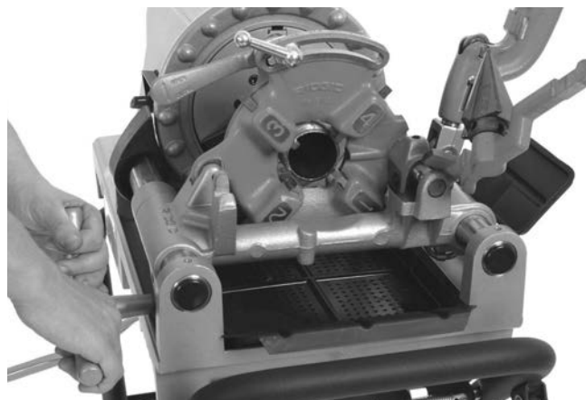
24-сурет – Кесу құбыры (811-А Жылдам ашылатын бастиек көрсетілген)
