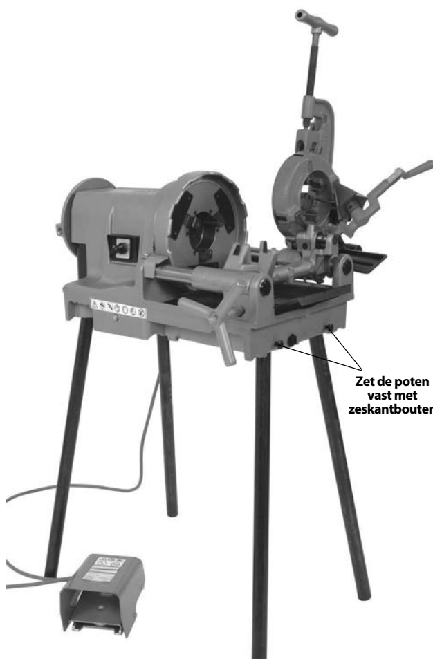
Afbeelding 4 – Schroefdraadsnijmachine gemonteerd op buispoten
