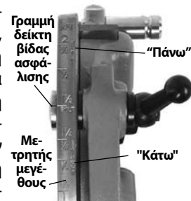
Εικόνα 13 – Ρύθμιση μεγέθους σπειρώματος
