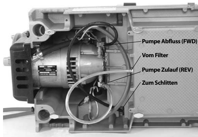
Abbildung 25B – Ölumpenanschlüsse für das Schneiden von Rechtsgewinden (Schalter auf FWD)
