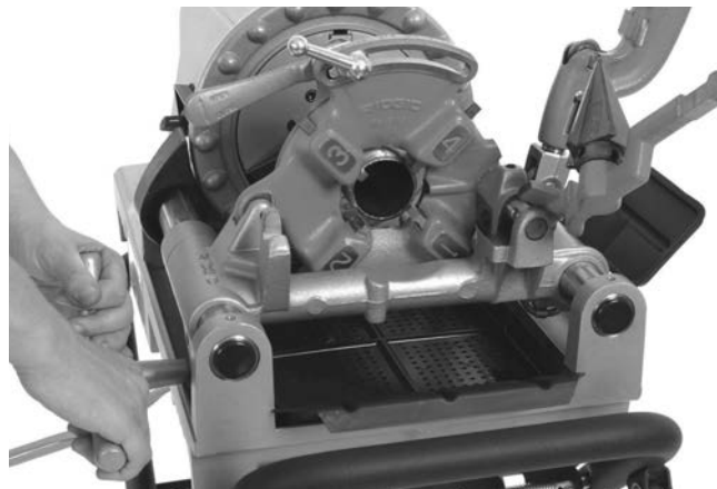
Obrázek 24 – Řezání závitu trubky (je zobrazena rychle otevírací závitorezná hlava 811-A)
