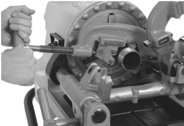
Figura 22 – Tăiere țeavă cu tăietorul
