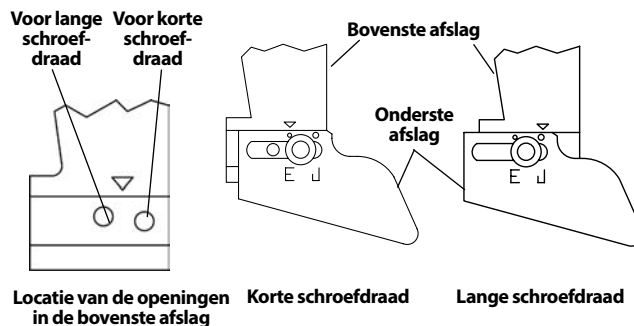
Afbeelding 18 – Bijstellen van de schroefdraadlengte
