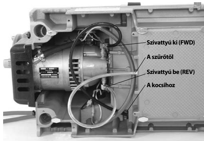
25B Ábra – Az olajszivattyú csatlakozásai jobbmenetnek (A kapcsoló FWD állásban)
