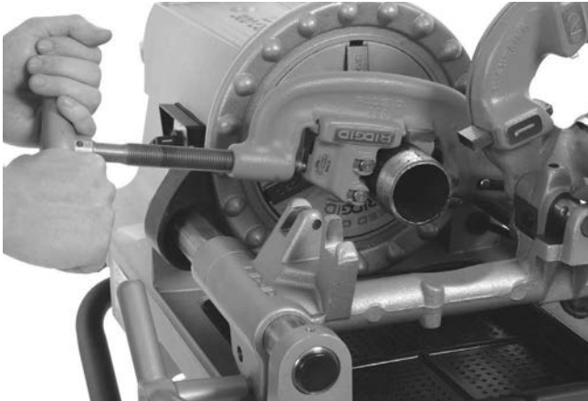
Εικόνα 22 – Κοπή σωλήνα με κόφτη
