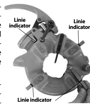
Figura 12 – Inserare filiere
