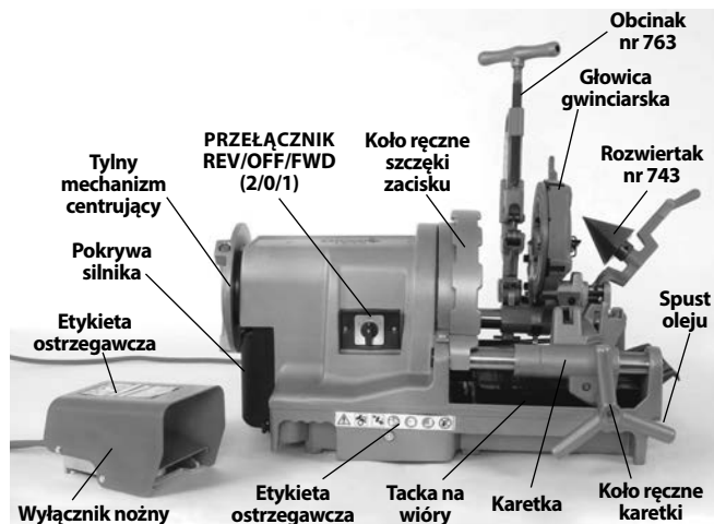
Rys. 2 – Gwintownica 1233
