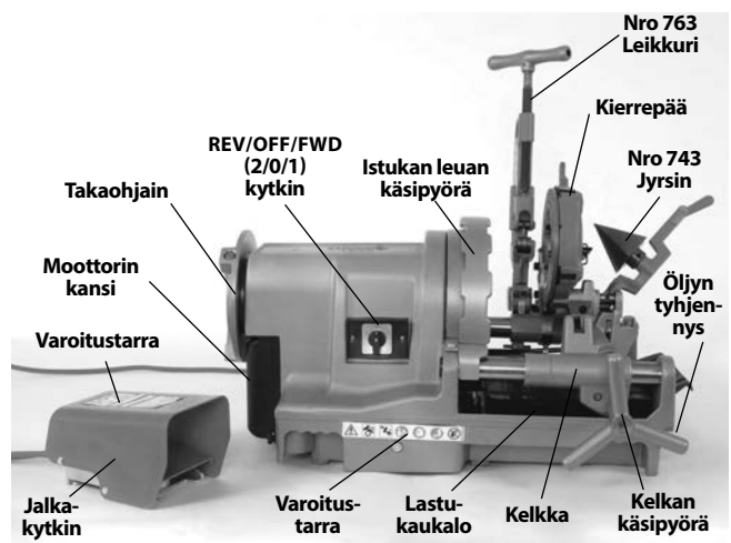
Kuva 2 – 1233-kierteityskone
