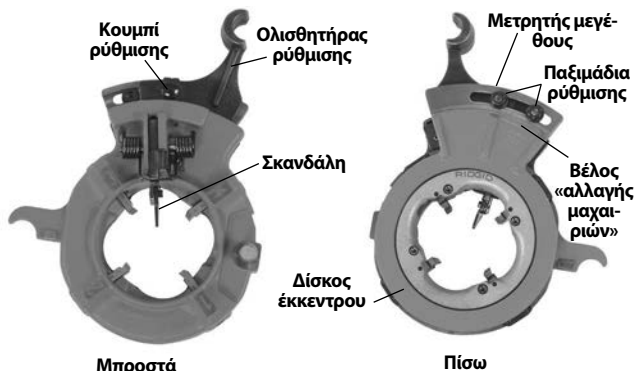
Εικόνα 15 – Φιλιέρα αυτόματου ανοίγματος με ανάσχυση
