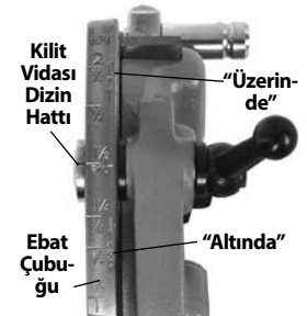
Şekil 13 – Diş Boyutunun Ayarlanması
