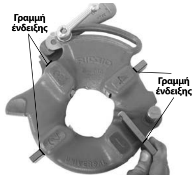
Εικόνα 8 – Τοποθέτηση μαχαiriών
