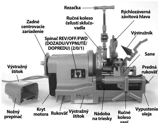
Obrázok 1 – Závítorez 300 Compact
