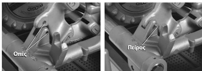
Εικόνα 26 – Διατήρηση φιλιέρας αριστερού σπειρώματος στη θέση της
