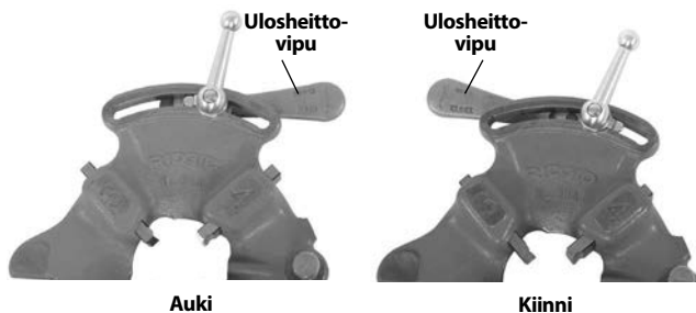
Kuva 7 – Vivun auki/kiinni-asento
