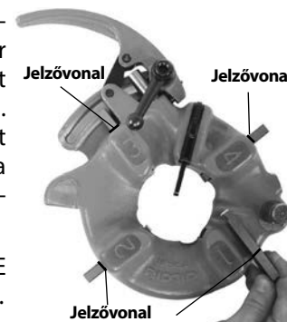
12. Ábra – Betétek behelyezése
