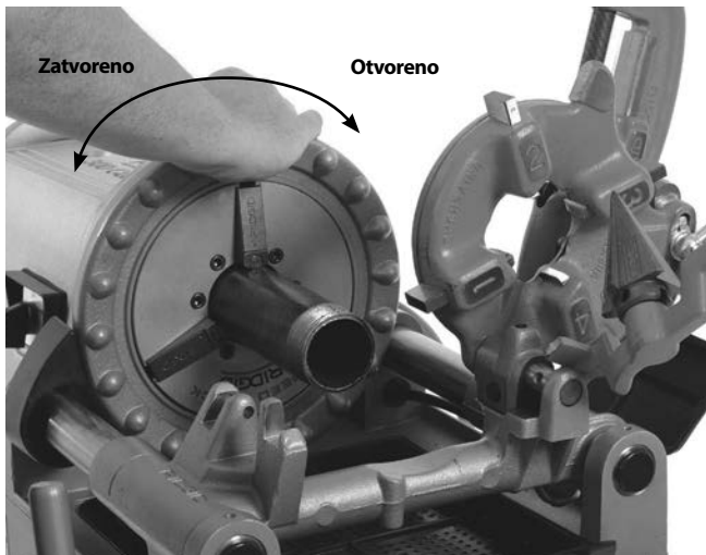
Slika 20 – Narezivanje cijevi
