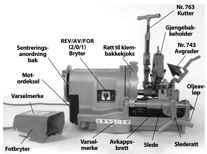
Figur 2 – 1233 Gjengemaskin
