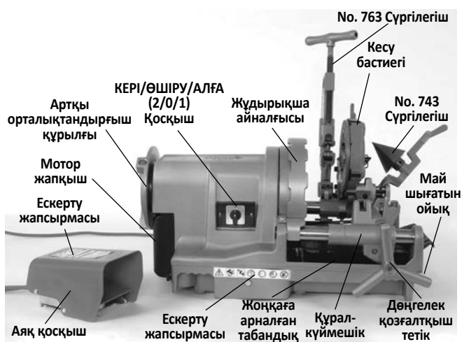
2-сурет – 1233 бұрандакесу құрылғысы
