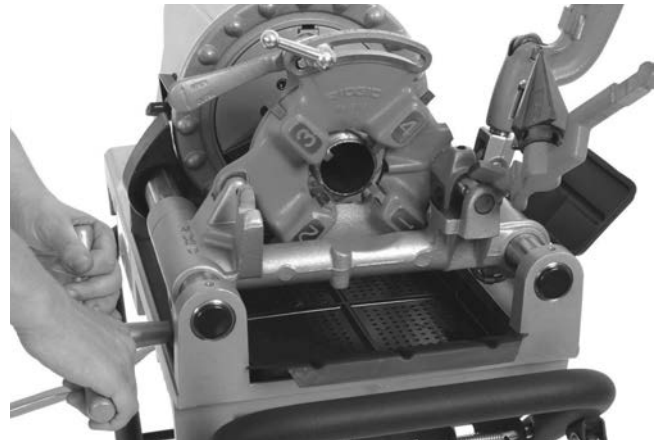
Figura 24 – Filetare țevi (811-este reprezentat un cap-filieră cu deschidere rapidă)
