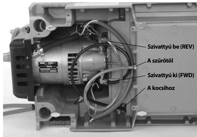
25A Ábra – Az olajszivattyú csatlakozásai balmenetnek (A kapcsoló REV állásban)
