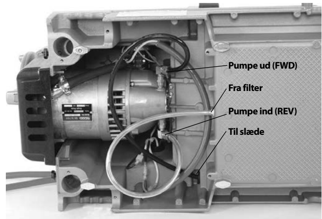
Figur 25B – Oliepumpetilslutninger for højrevindskæring (kontakt i stillingen FWD)
