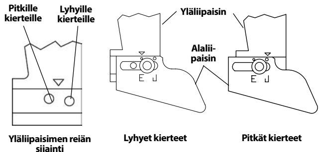
Kuva 18 – Kierteen pituuden säätäminen
