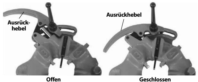
Abbildung 11 – Geöffnete/geschlossene Position
