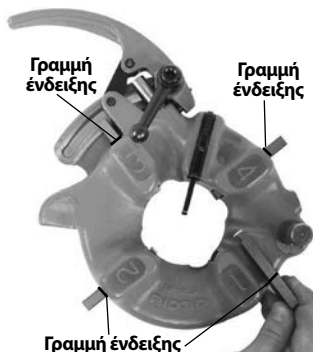
Εικόνα 12 – Τοποθέτηση μαχαιριών
