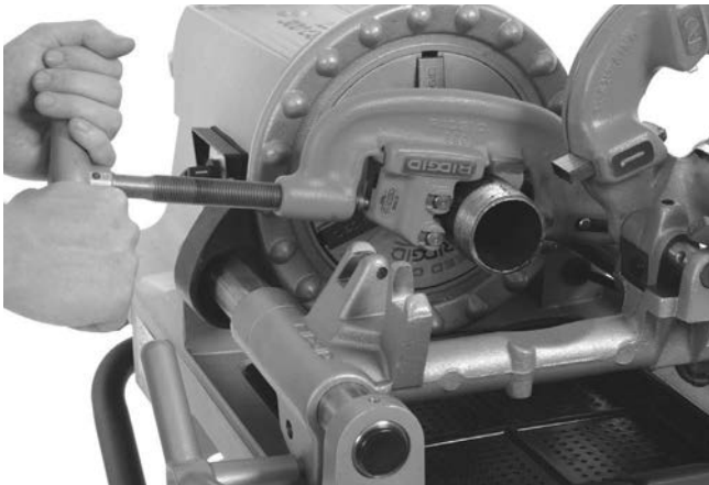
Abbildung 22 – Schneiden eines Rohrs mit dem Rohrabschneider
