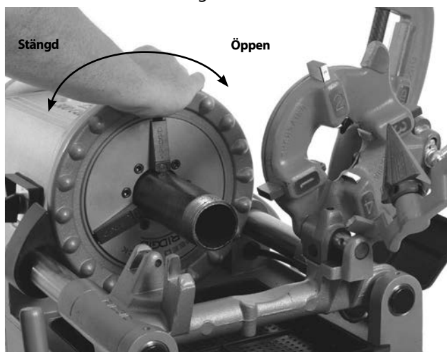
Figur 20 – Chucka rör
