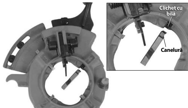
Figura 16 – Inserare cuțite-filieră
