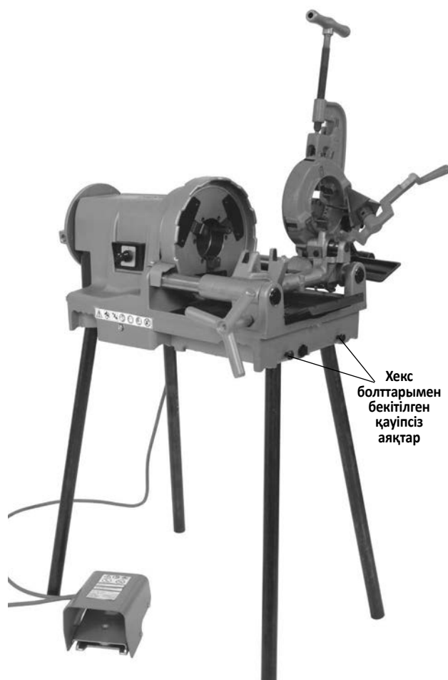
4-сурет – Құбыр аяқтарына орнатылған бұрандакесу құрылғысы
