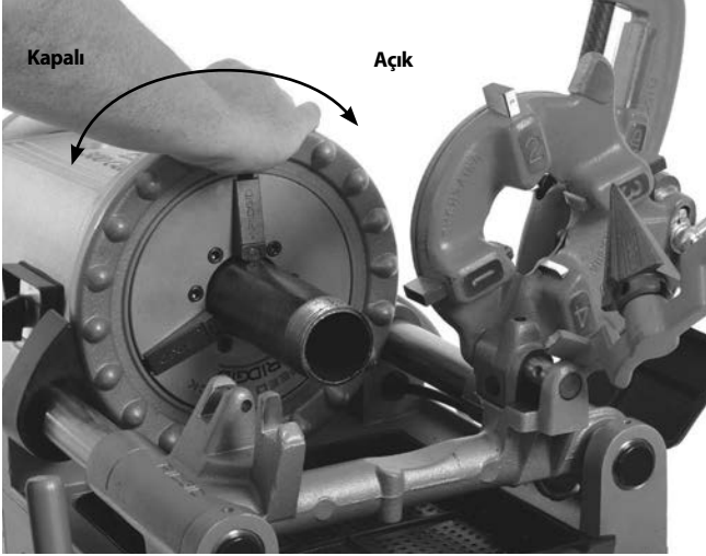
Şekil 20 – Mandren Boru
