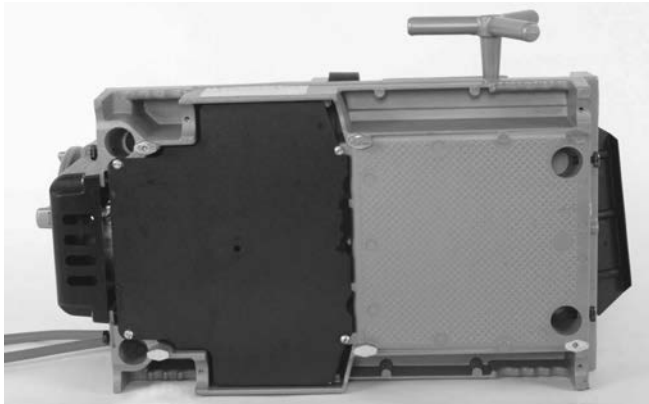
Abbildung 25C – Abdeckung angebracht
