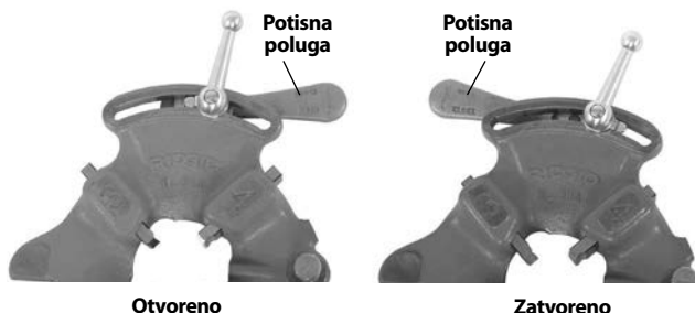
Slika 7 – Pozicija otvoreno/zatvoreno
