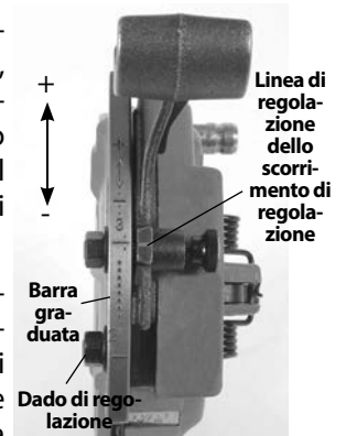
Figura 17 – Regolazione della dimensione della filettatura
