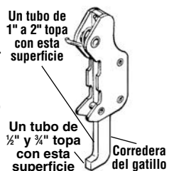
Figura 14 – Posición del gatillo
