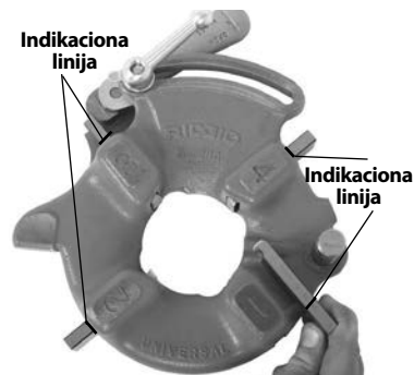
Slika 8 – Postavljanje noževa
