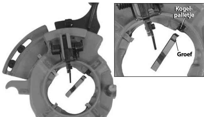
Afbeelding 16 – Aanbrengen van de snijkussens
