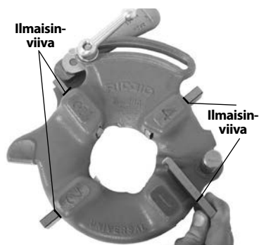
Kuva 8 – Terien asentaminen
