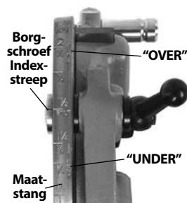
Afbeelding 13 – Schroefdraadmaatinstelling
