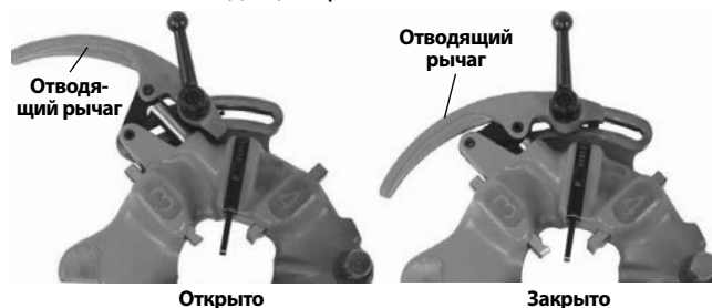
Рис. 11 – Открытое/закрытое положение
