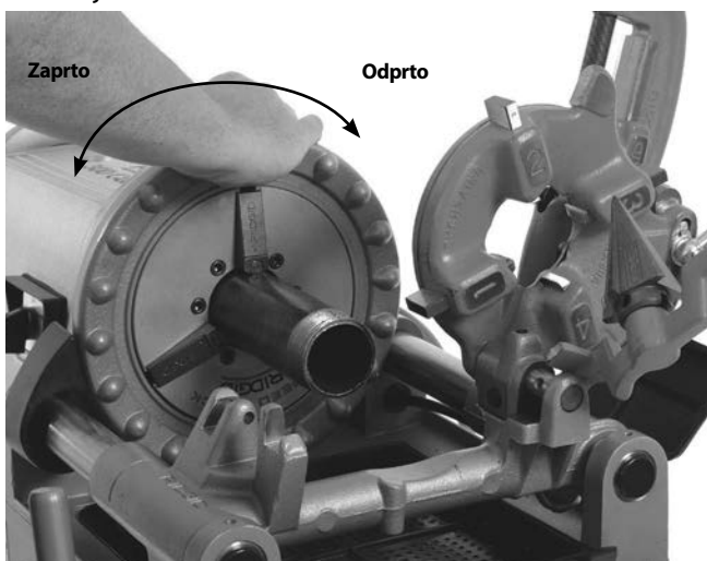
Slika 20 – Cev glave
