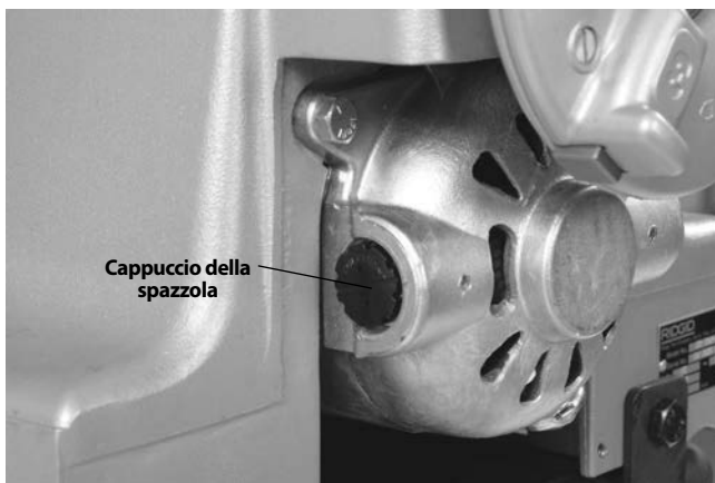
Figura 32 – Rimozione del coperchio del motore/ Sostituzione delle spazzole
