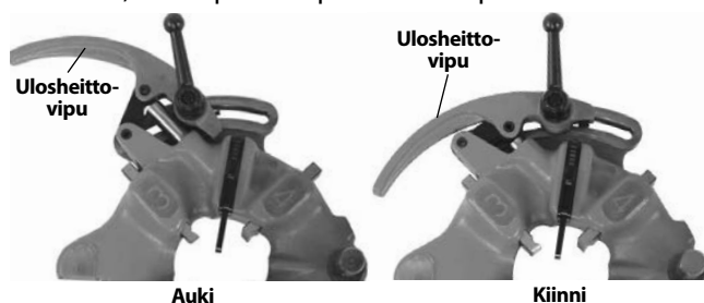
Kuva 11 – Auki/kiinni-asento
