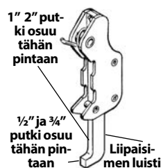
Kuva 14 – Liipaisimen luistin säätäminen
