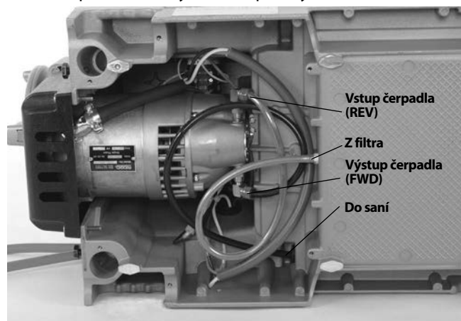
Obrázok 25A – Pripojenia olejového čerpadla pre rezanie ľavého závitú (spínač v polohe REV)
