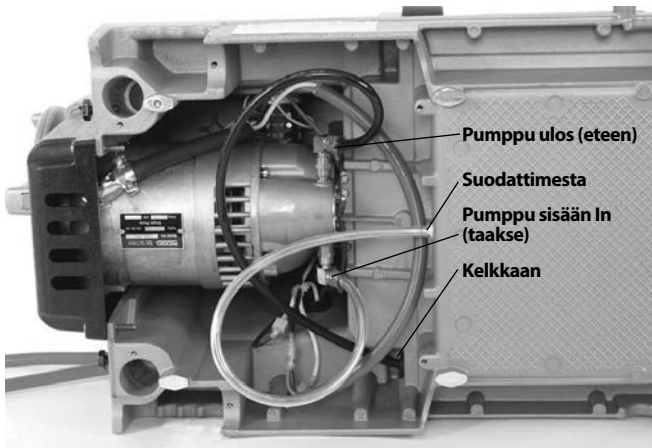
Kuva 25B – Öljypumpun liittämät oikeakätiseen kierteitykseen (kytkin asennossa FWD (eteen))
