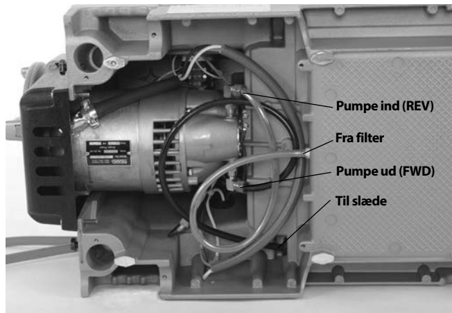
Figur 25A – Oliepumpetilslutninger for venstrevindskæring (kontakt i stillingen REV)
