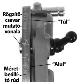
13. Ábra – A menet méretének beállítása
