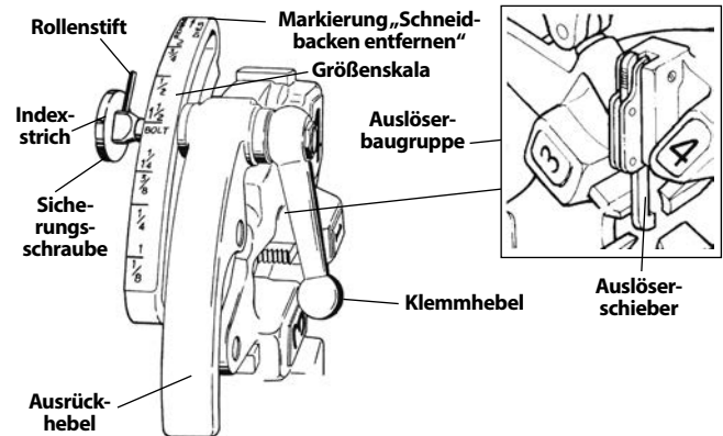
Abbildung 10 – Selbstöffnender Universalschneidkopf
