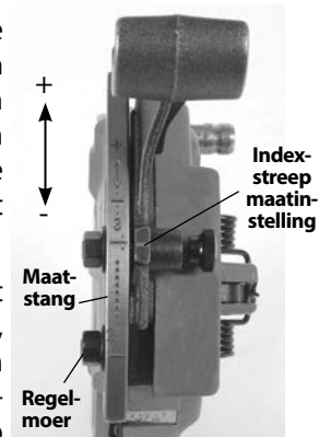
Afbeelding 17 – Schroefdraadmaatinstelling
