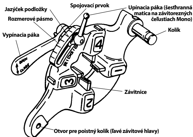
Obrázok 6 – Rýchlozáverná závitová hlava
