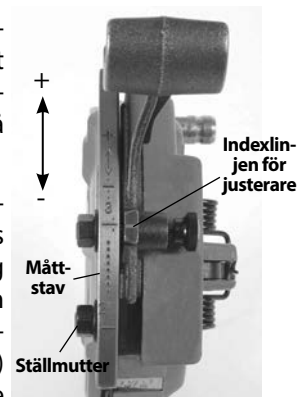
Figur 17 – Justera gängdimension
