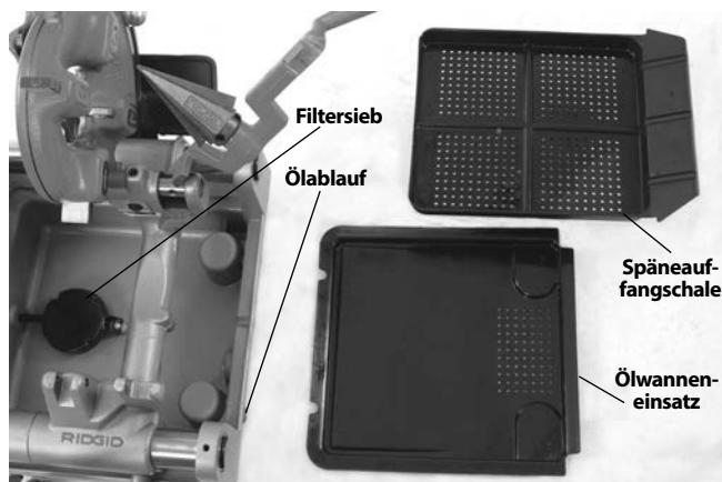
Abbildung 30 – Filtersiebbaugruppe
