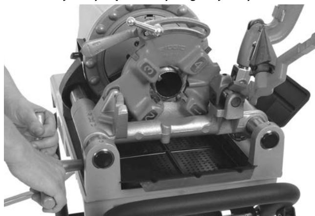
Rys. 24 – Gwintowanie rury (pokazano szybkoobrotową głowicę gwinciarzką 811-A)
