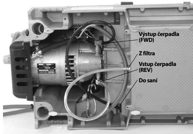
Obrázok 25B – Pripojenia olejového čerpadla pre rezanie pravého závitú (spínač v polohe FWD)
