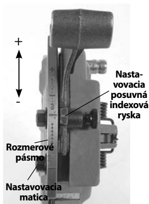
Obrázok 17 – Nastavenie veľkosti závitov
