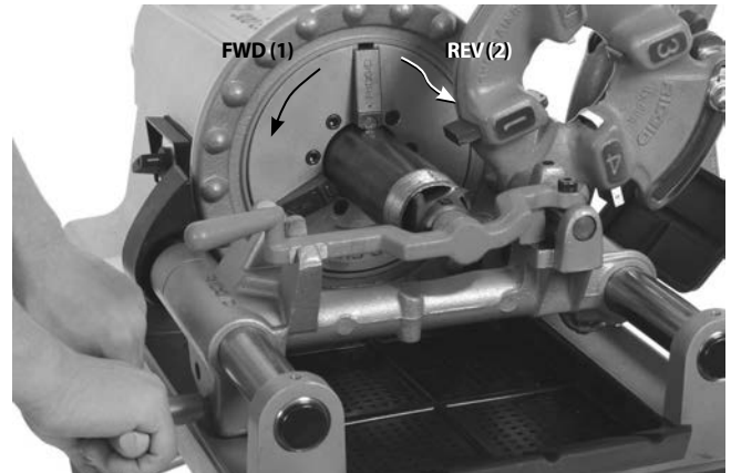
Obrázok 23 – Vystruhovanie rúry pomocou výstružníka, otáčanie stroja
