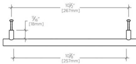
TOP VIEW SCALE: 3"=1'-0"
