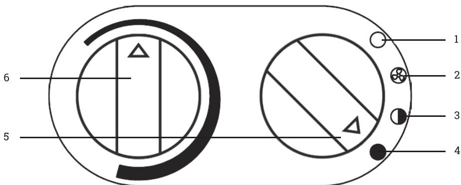
Рис. 2. Панель управления: 1) положение выключения прибора, 2) положение режима вентиляции без нагрева, 3) положение частичной мощности нагрева, 4) положение полной мощности нагрева, 5) ручка переключателя режимов, 6) ручка регулировки термостата
