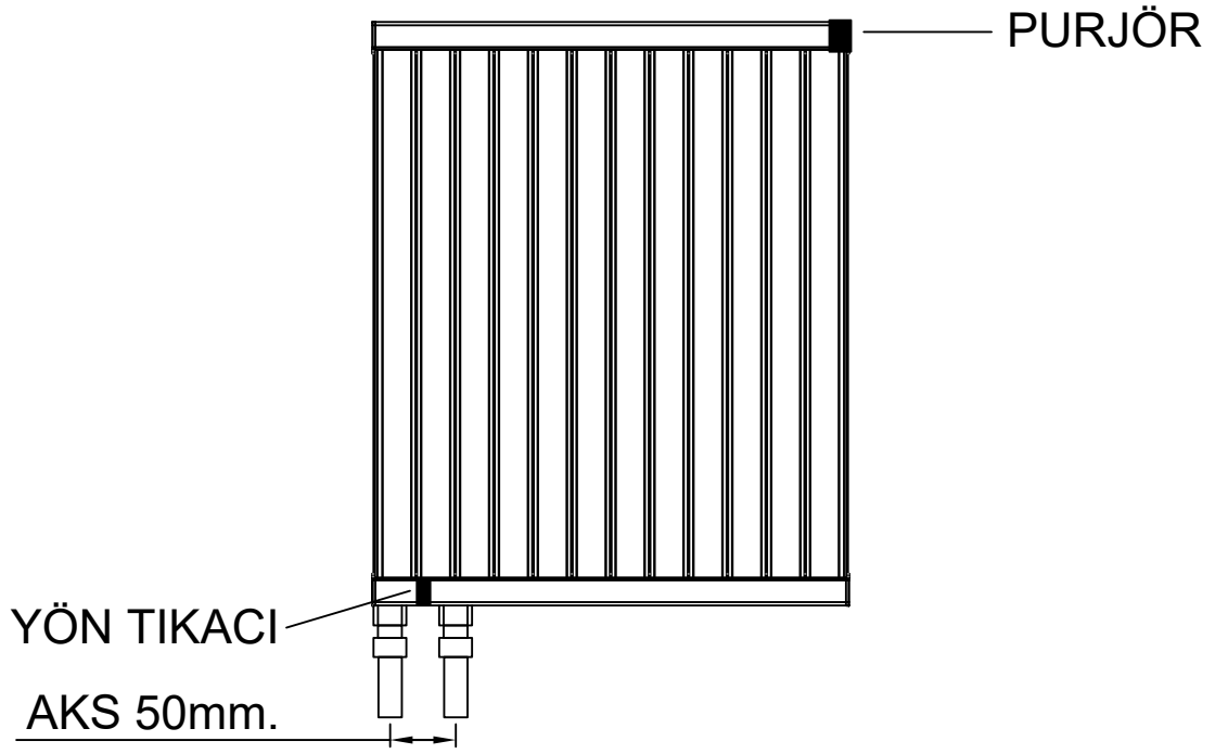
BELLA RADYATÖR KONPAKT BAĞLANTI GÖRÜNTÜSÜ
