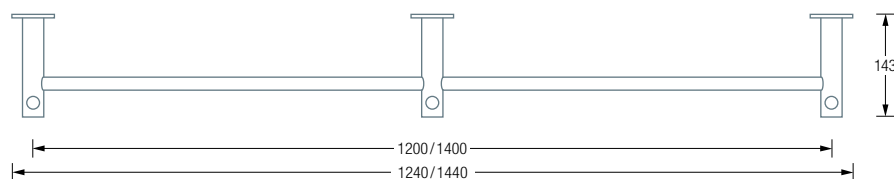
G4-1200 / 1400 Draufsicht:
