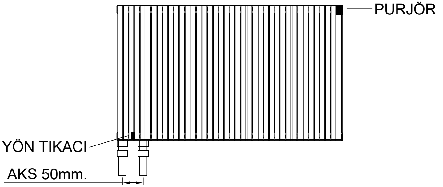
FELICE RADYATÖR KOMPAKT BAĞLANTI GÖRÜNTÜSÜ
