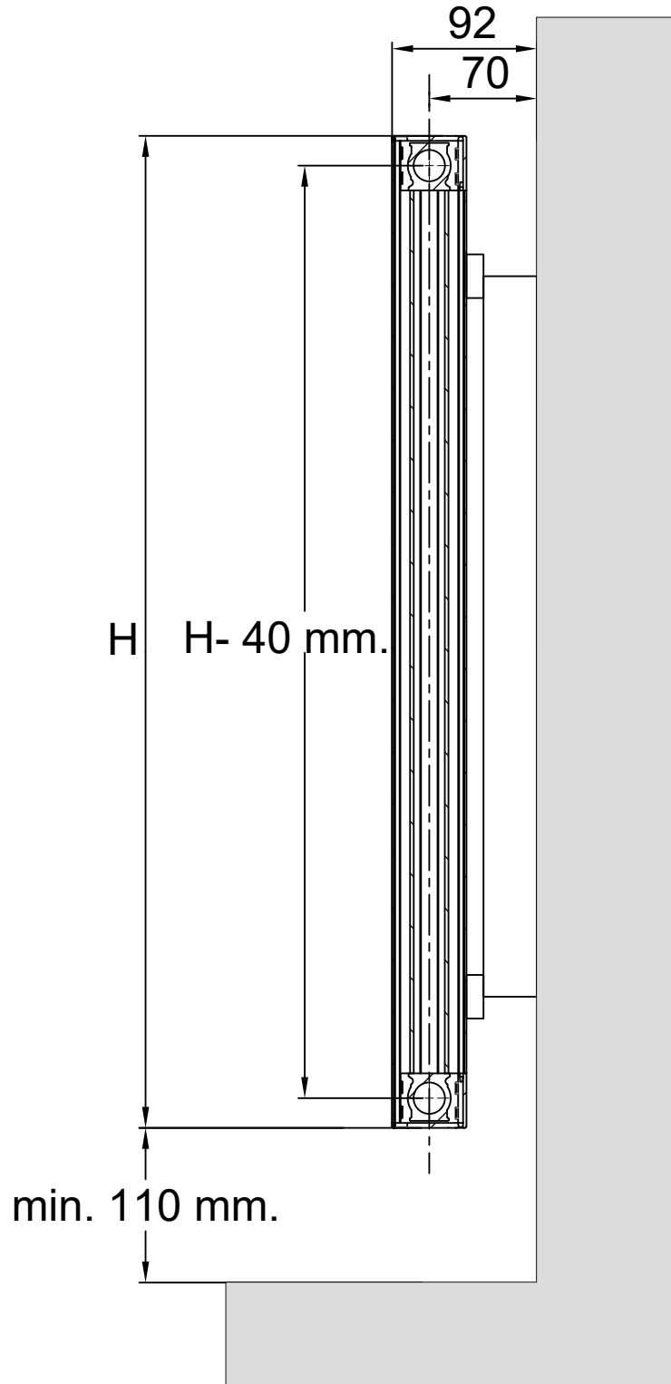
FELICE RADYATÖR DUVAR MONTAJ GÖRÜNTÜSÜ
