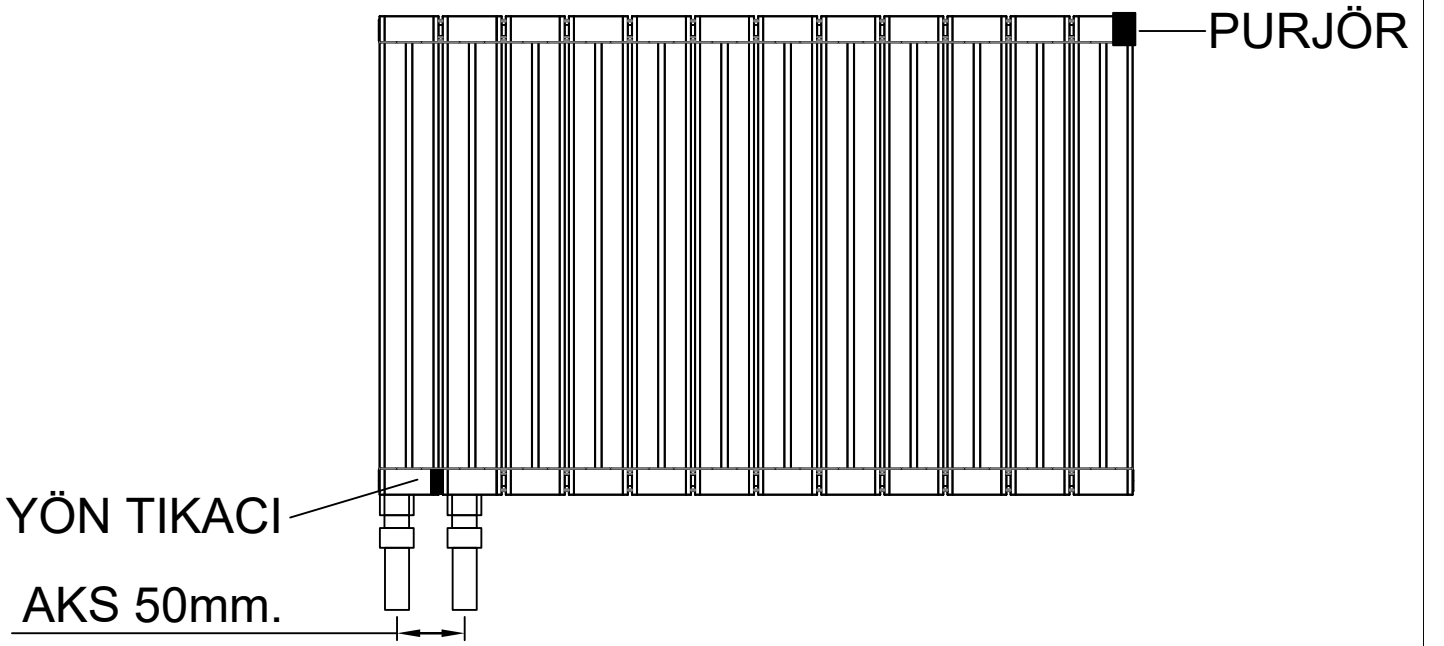
RAFFINATO RADYATÖR KOMPAKT BAĞLANTI GÖRÜNTÜSÜ
