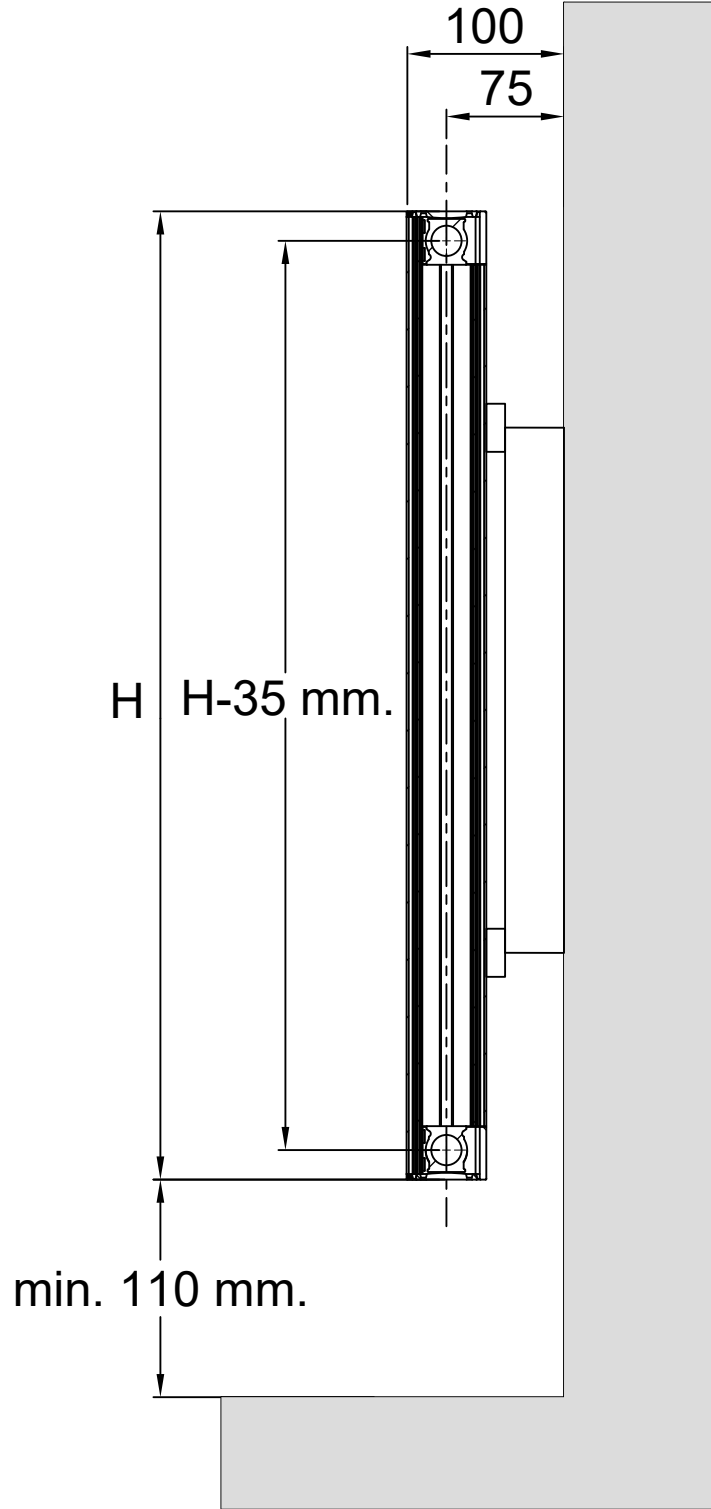
RAFFINATO RADYATÖR DUVAR MONTAJ GÖRÜNTÜSÜ
