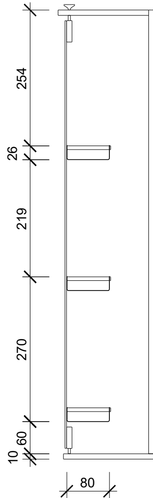
Seitenansicht side view
