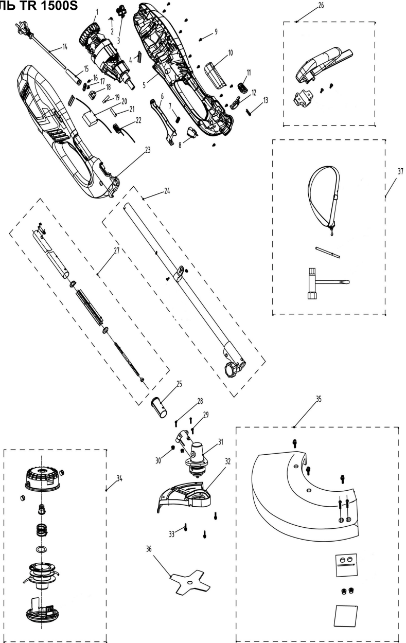
Рис. 6. Схема частей
