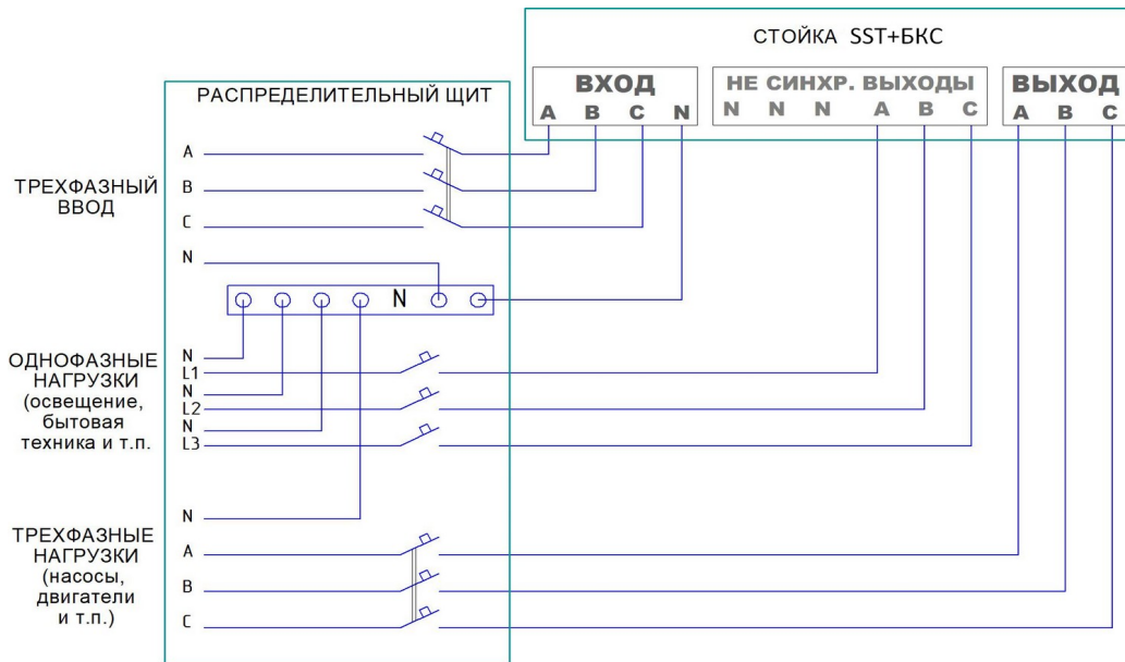
Рисунок 1. Рекомендуемая схема подключения Стойки SST+БКС к сети.
