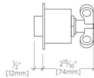
SIDE VIEW SCALE: 3"=1'-0"
