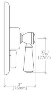
SIDE VIEW SCALE: 3"=1'-0"
