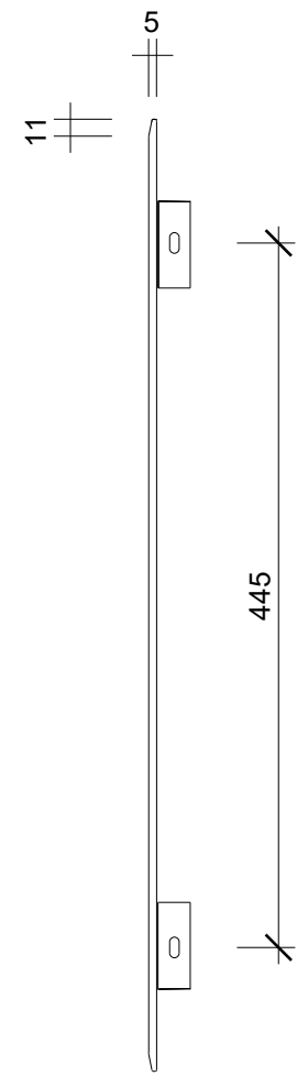
Seitenansicht side view
