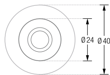
HG24-25HS-B Draufsicht:
