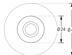
HG24-50K45-B Draufsicht:
