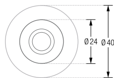
HG24-25K40-B Draufsicht:
