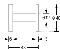
HA1-R40S40-B Seitenansicht:
