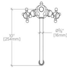
TOP VIEW SCALE: 1 1/2"=1'-0"
