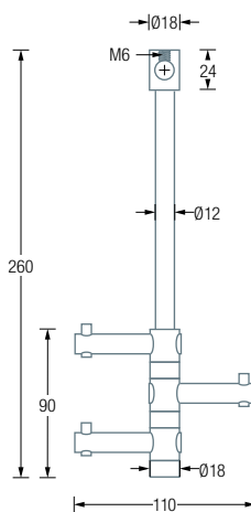
T3F Seitenansicht:
