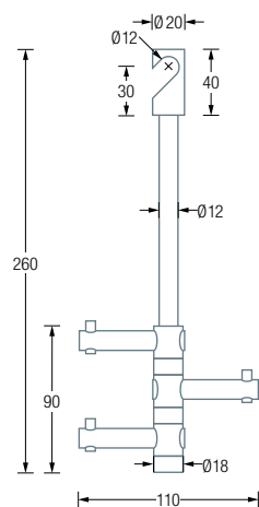
T3H Seitenansicht:
