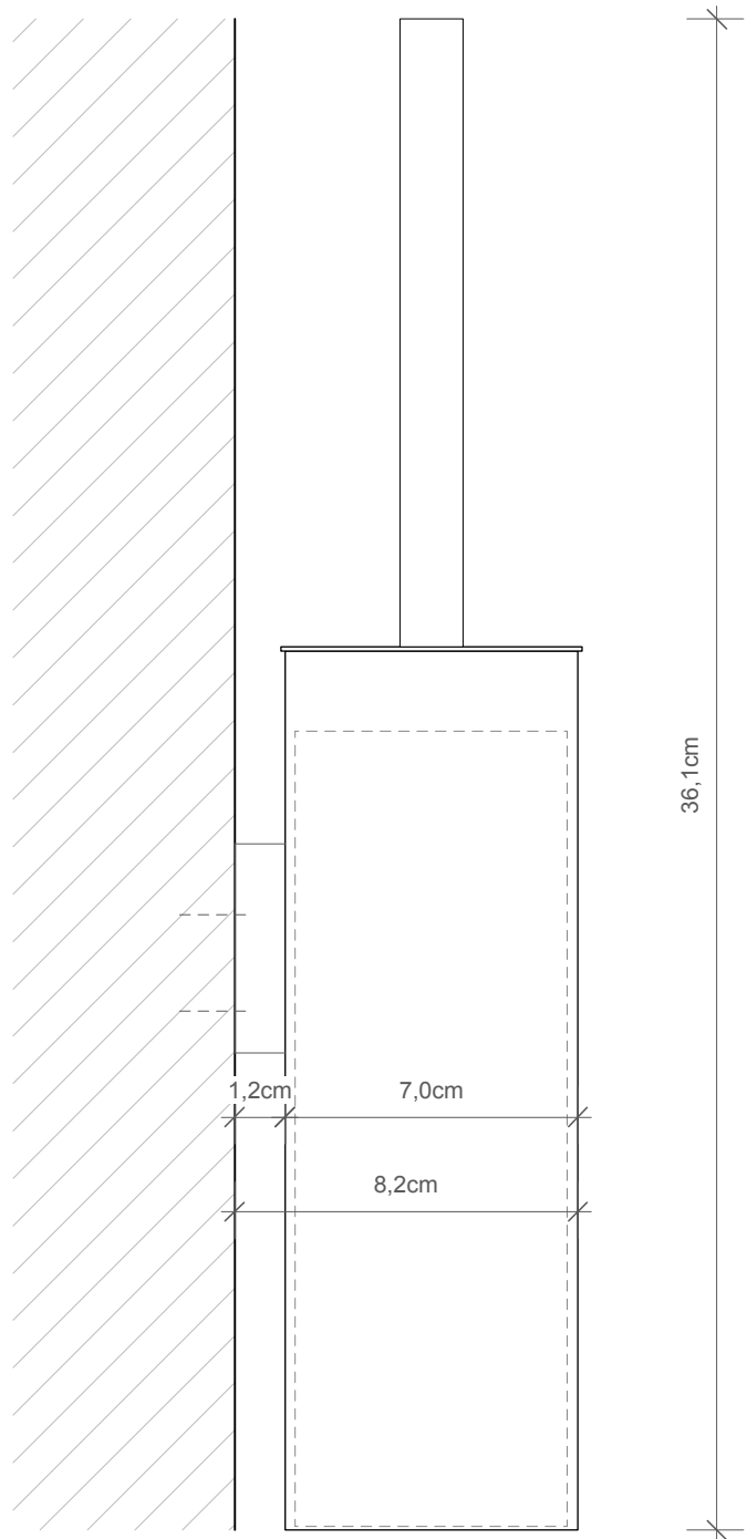
Seitenansicht Side View
