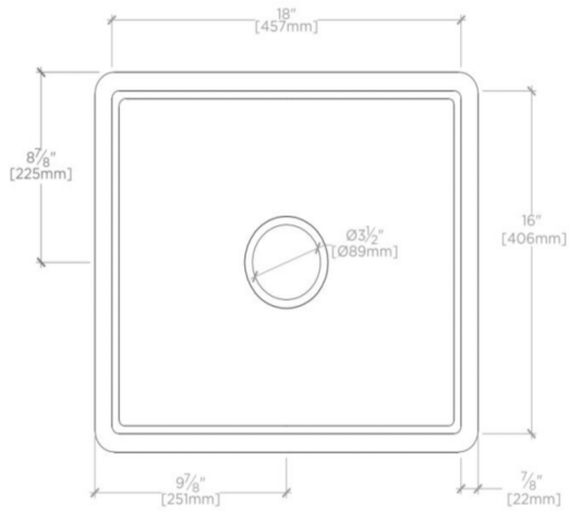
TOP VIEW SCALE: 1/2"=1'-0"
