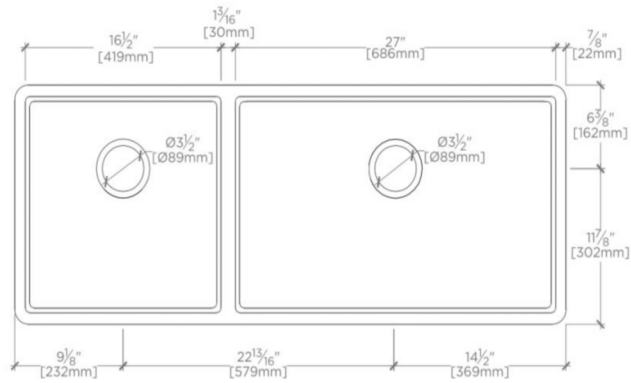
TOP VIEW SCALE: 1"=1'-0"
