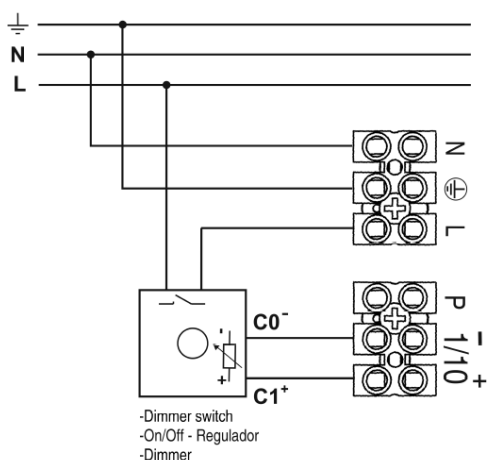
REGULACIÓN MEDIANTE SISTEMA 1-10 V Diagrama X
