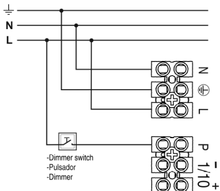
REGULACIÓN MEDIANTE PULSADOR Diagrama Y
