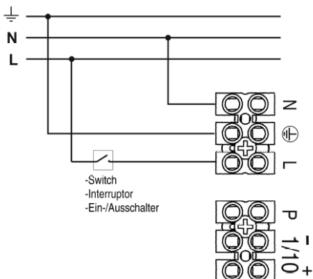
SIN REGULACIÓN Diagrama Z
