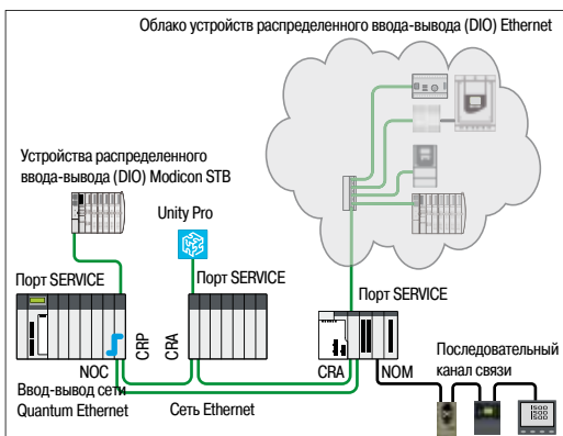
Подключение к порту SERVICE
