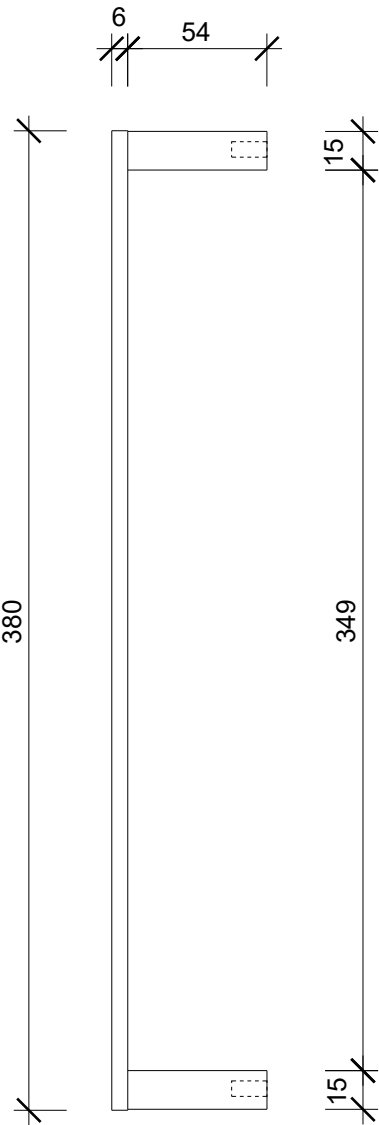
Seitenansicht side view
