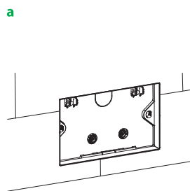
Вар. 2 Установка клавиши на инсталляцию Unifix UNI0000i32
