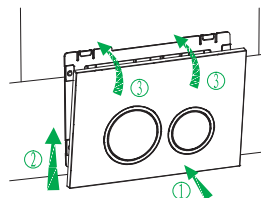
Вар. 2 UNI0000i32 Unifix құрылғысына клавишаны орнату
