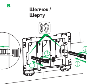
Вар. 2 UNI0000i32 Unifix құрылғысына клавишаны орнату
