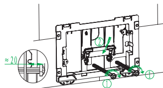
Вар. 2 Установка клавиши на инсталляцию Unifix UNI0000i32
