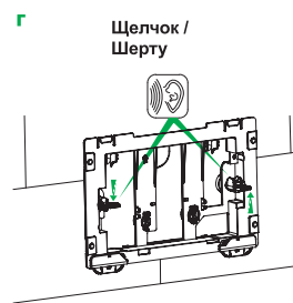
Вар. 2 UNI0000i32 Unifix құрылғысына клавишаны орнату
