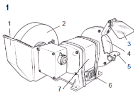
Рис.1 Общий вид станка
