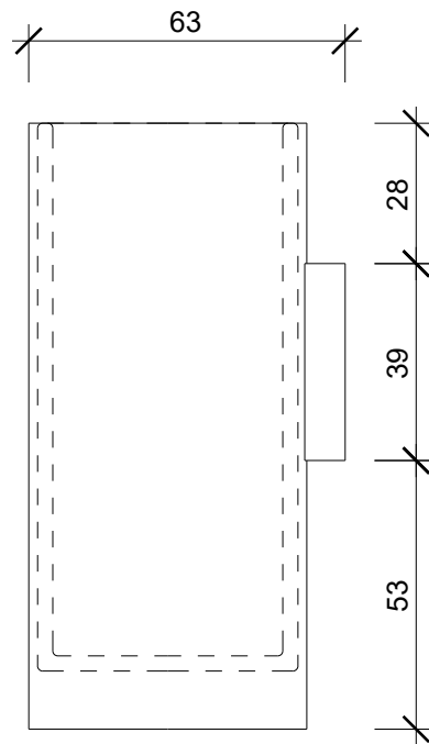
Seitenansicht side view
