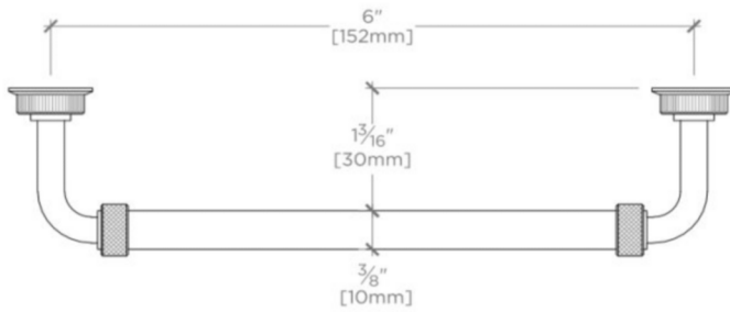
TOP VIEW SCALE: 6"=1'-0"
