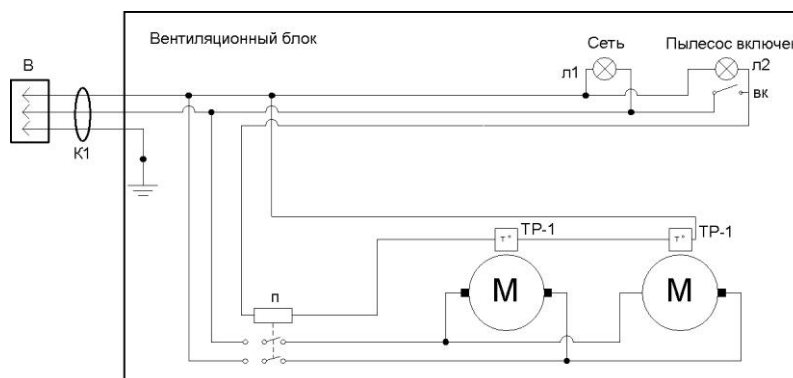
Рис. 3 Схема электрическая принципиальная
